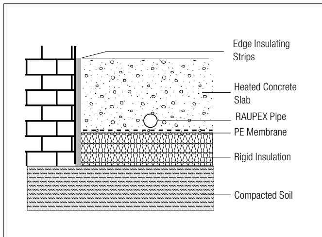
Fig. 5.1: Edge joint
